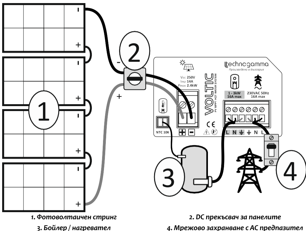
3. Бойлер / нагревател
